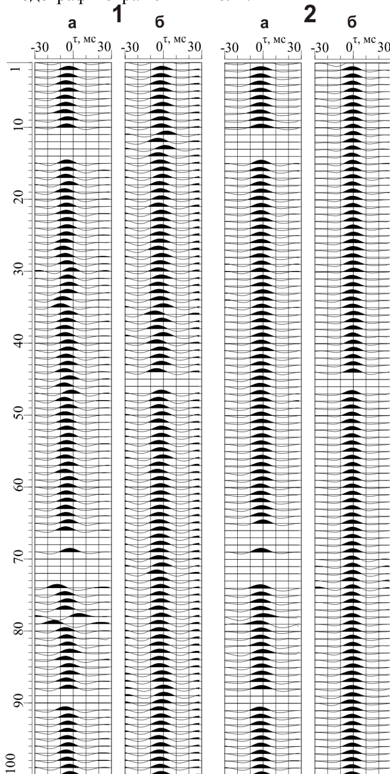
Рис. 1 Коррекция статических поправок «Поликор». 1 – Ряды корреляционных функций до коррекции, 2 – ряды корреляционных функций после коррекции. а – ряды корреляционных функций по пунктам возбуждения, б – ряды корреляционных функций по пунктам приема.
