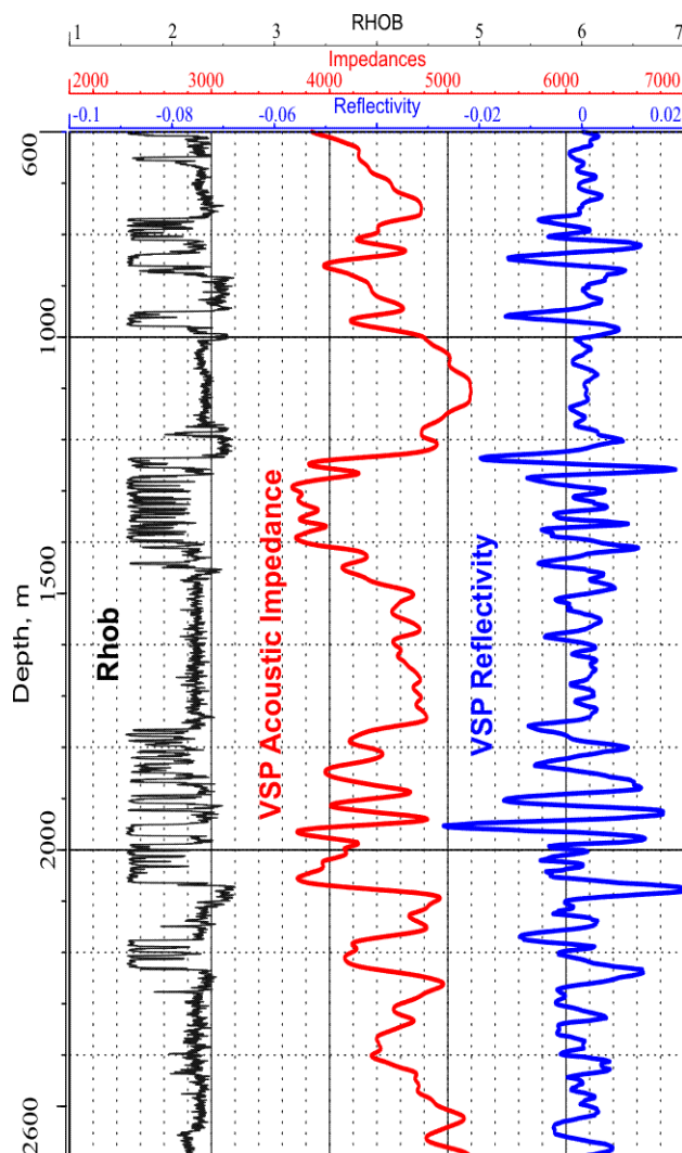
Fig. 3. VSP-log tie
