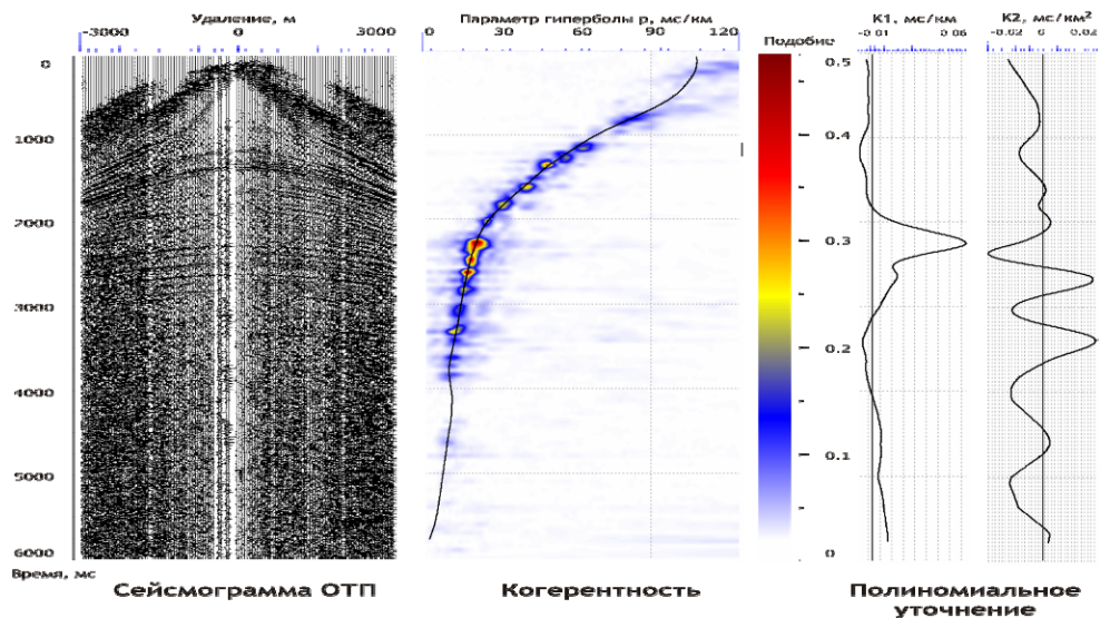
Рис. 2. Сейсмограмма ОТП, спектр когерентности и кривые кинематических параметров отраженных волн.
