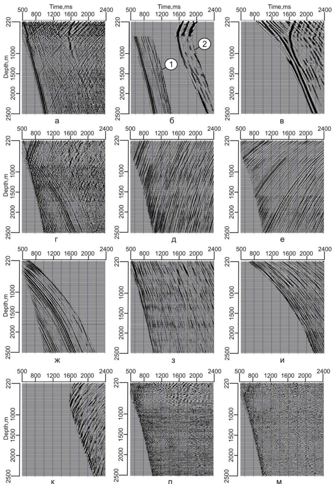
Рис.3. Результаты селекции реальных данных НВСП (Западная Сибирь): а) Р-компонента исходного волнового поля, б) прямые волны: продольная (1) и поперечная (2), выделенные из Р компоненты, в) наложение двух видов прямой S-волны, выделенных из R-компоненты исходного поля (рис.2а) г) Z-компонента исходного поля после вычитания прямых волн д)-к) волновые поля после селекции из Z-компоненты: отраженной продольной (DPUP), отраженной обменной поперечной (DPUS) (из Y компоненты), обменной падающей (DPDS), кратной
